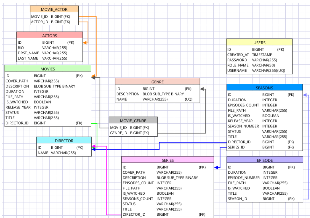
Рисунок 6 – ER-диаграмма
